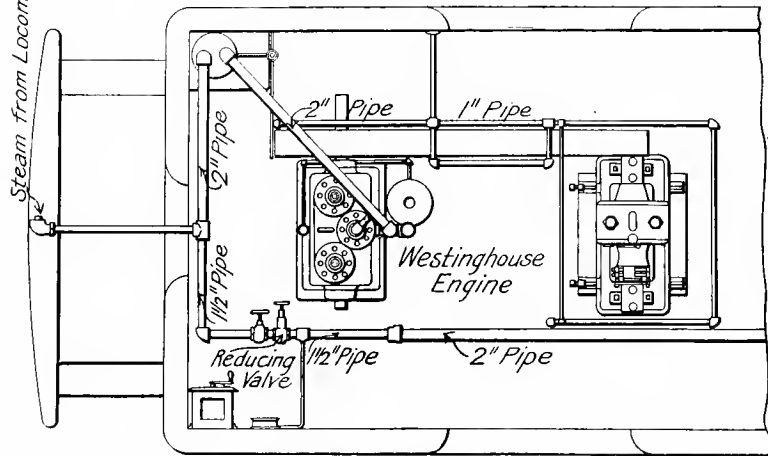
Fig. 594. Part Plan.
